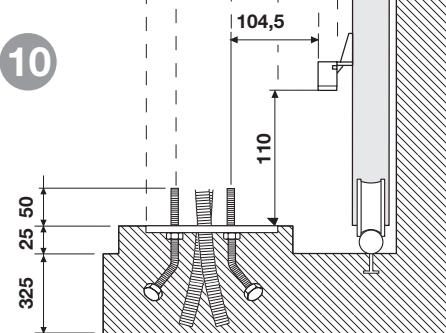
ANCORAGE DU MOTORÉDUCTEUR vue latérale
